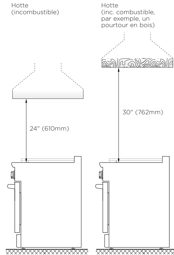
Installation en îlot
