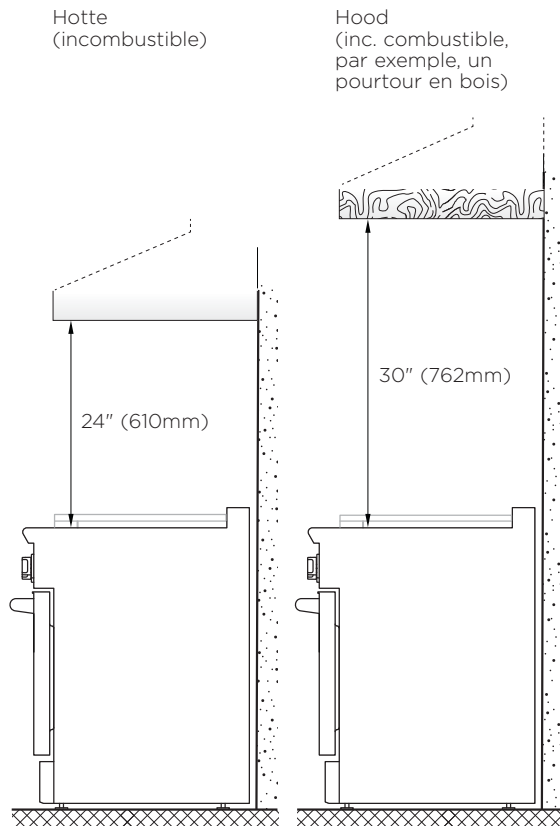
Installation au mur
